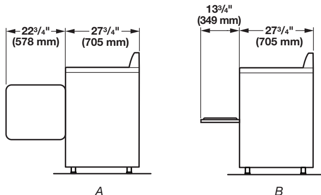
A. Porte à grande ouverture latérale B. Porte rabattable à large ouverture
